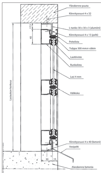
Kiinteän 1-lasisen seinän asennus L-listalla
