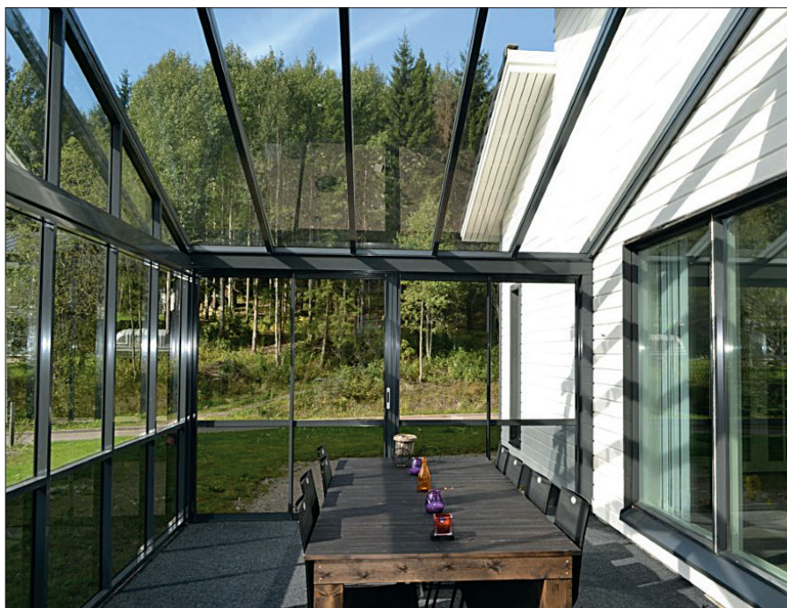
Kiinteän 1-lasisen seinän asennus L-listalla
